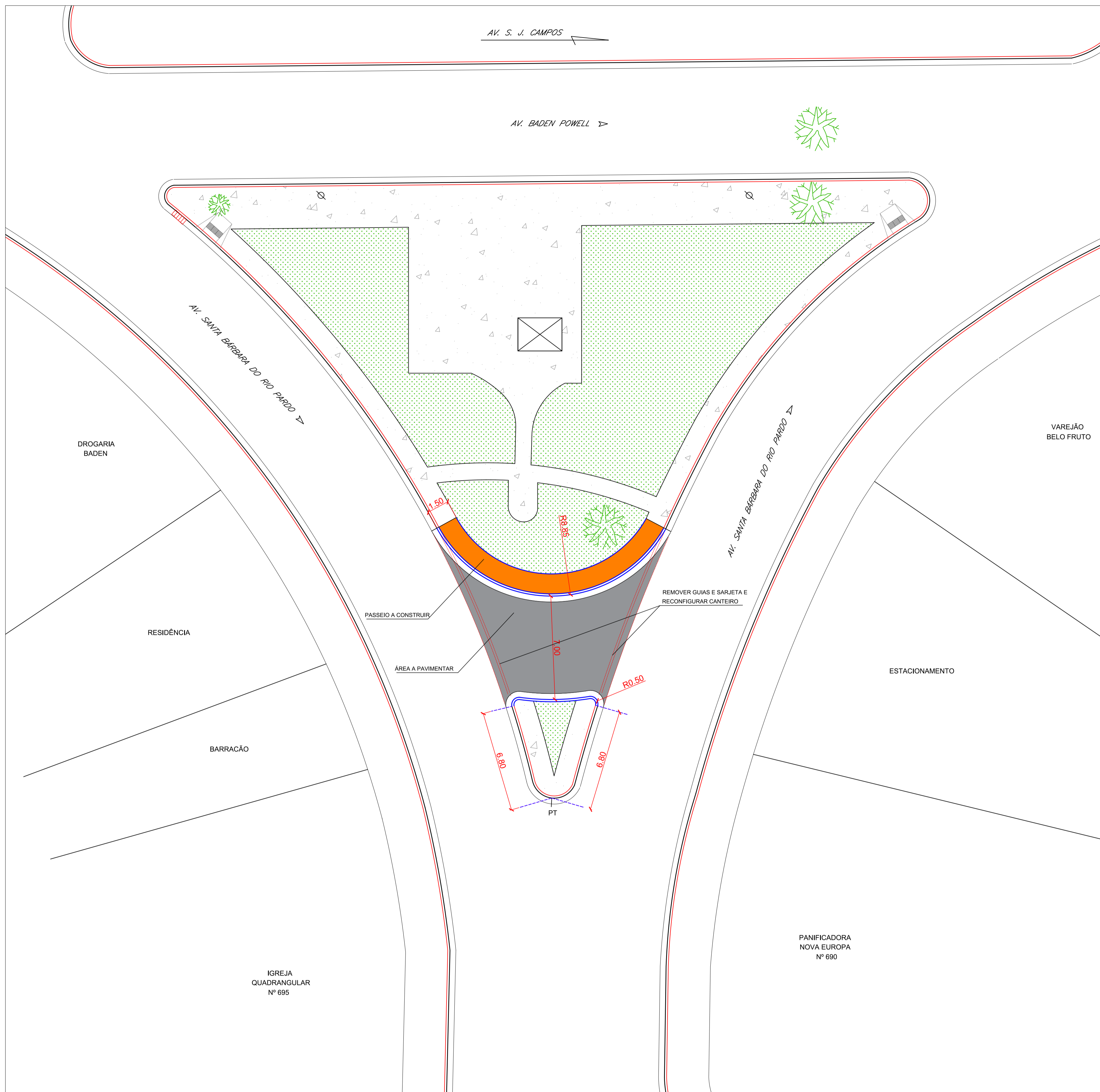
↑ PLANTA BAIXA - IMPLANTAÇÃO esc. 1:150
